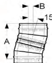
Fig. Coude 30°
