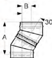
Fig. Coude 45°
