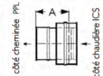
Raccord de jonction ICS sur PPL
