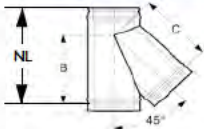
Raccord de conduite de cheminée 45° avec blocage anti-condensat
