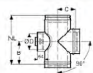
Raccord de conduite de cheminée 90° avec raccordement trappe de ramonage, pour mazout et gaz
