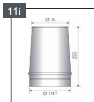
Finition conique
