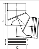
Coude 85° avec pied de support
