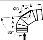
Coude 85° avec trappe de visite, pour combustibles solides
