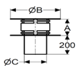
Chapeau antipluie Anti-splash (avec grille)
